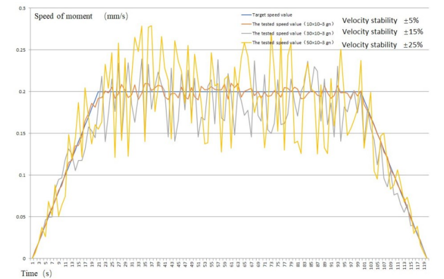
Fig. 4 Analysis results in discrete time sequence 图4 干涉系统速度在不同时刻分析结果
