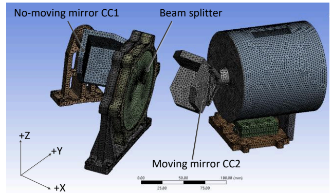
Fig. 2 Finite element model of the interferometer 图2 干涉系统有限元模型示意图
