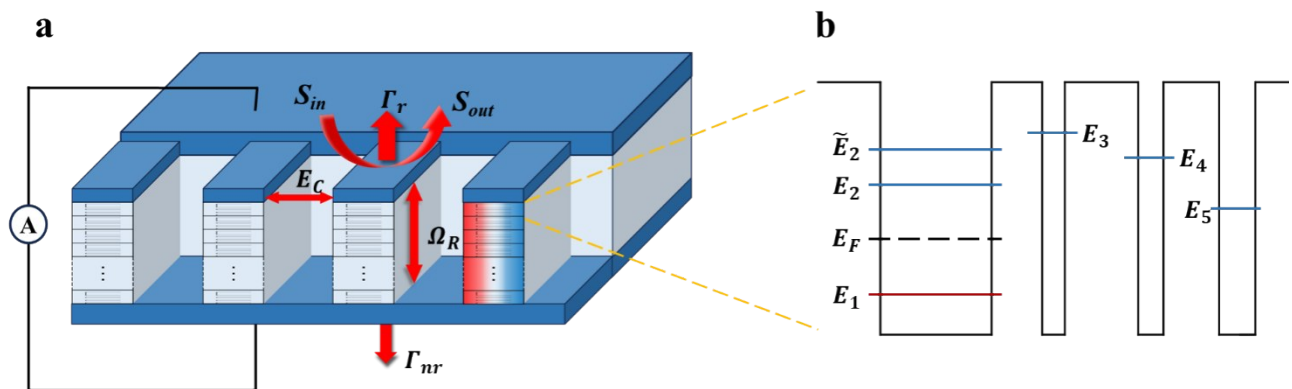
图1 谐振腔光电探测器装置与能级分布示意图。(a) 装置示意图:输入光场 S_{in} 和输出光场 S_{out} 。辐射耗散系数 \Gamma_r 和非辐射耗散系数 \Gamma_{nr} ,腔模电场 E_c 和真空拉比频率 \Omega_R 。(b) 能级分布示意图:基础能级 E_1 、第一激发态 E_2 、集体激发电子能级 \widetilde{E}_2 、费米能级 E_F 和提取能级 E_3 。
