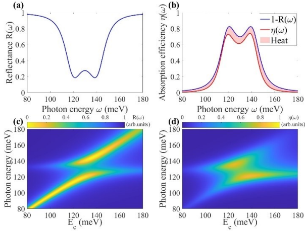
图2 光电探测器的反射率和吸收效率。(a) 在 E_c = 130 meV, g = \Omega_R \approx 11 meV, \omega_{31} = 141 meV 条件下的反射谱线; (b) 在相同条件下的吸收率谱线, 着色部分为 \Delta(\omega) , 蓝色线为 1 - R(\omega) , 红色线为 \eta(\omega) ; (c) 改变腔模频率 E_c 计算得到的反射谱映射; (d) 改变腔模频率 E_c 计算得到的吸收率映射图。
