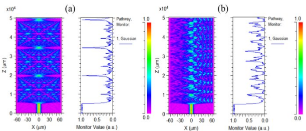
Fig. 2 Simulation of light field. : (a) Linear NCF; (b) Curved NCF 图2 光场模拟仿真图.: (a) 直线型 NCF; (b) 弯曲线型 NCF
