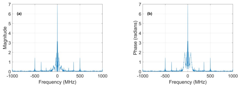
图4 最小值处仿真波形与GF-7波形的频域分析:(a)幅度差;(b)频谱差模
