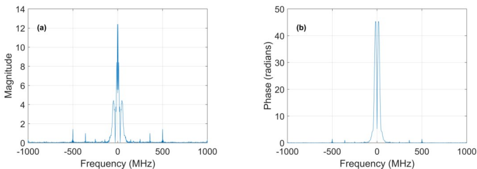
图7 最小值处仿真波形与GF-7波形的频域分析:(a)幅度差;(b)频谱差模
