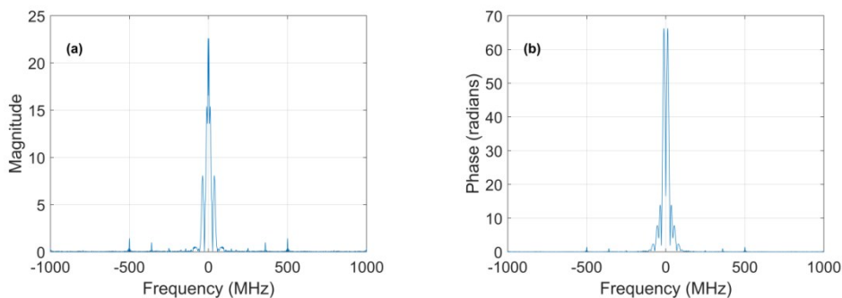
图5 任选仿真波形与GF-7波形的频域分析:(a)幅度差;(b)频谱差模
