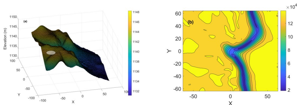
图 3 足印 142 号所在区域:(a) DEM;(b) 相关系数等高线
