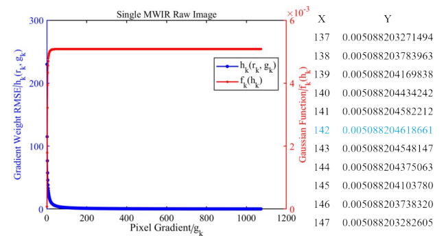
Fig. 7 Distribution curves of pixel gradient g_k corresponding to gradient weight RMSE h_k(r_k, g_k) and Gaussian function f_k(h_k) for a single MWIR raw image, and the computed optimal pixel gradient g_{opt} 图 7 单张中波红外原始图像的像素梯度 g_k 对应的梯度权重 RMSE h_k(r_k, g_k) 和高斯函数 f_k(h_k) , 以及计算的最佳像素梯度 g_{opt}
