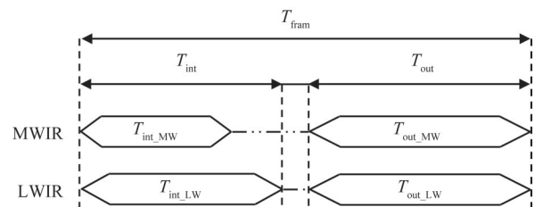
图5 积分-读出时序图
