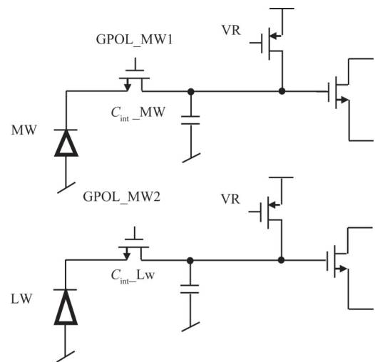
图4 双色读出电路输入级电路原理图
