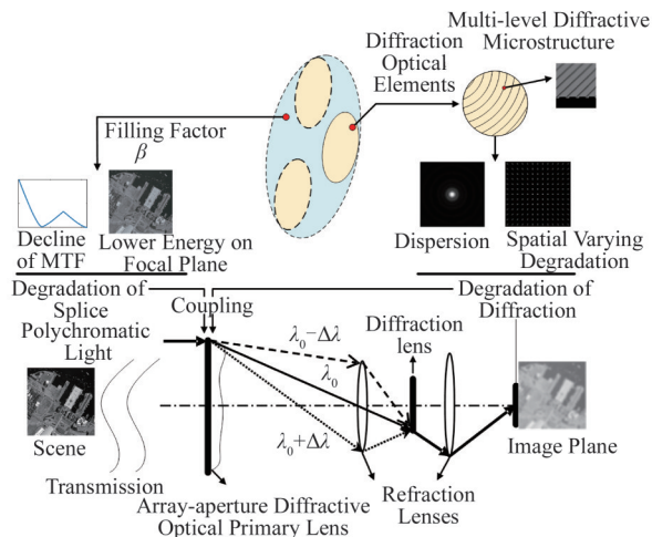
Fig. 1 Mechanism of degradation 图1 成像机理
