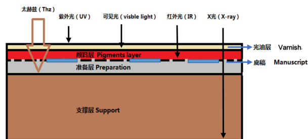
图7 常用电磁波穿透绘画作品厚度
