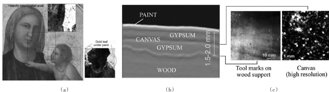
图9 太赫兹时域成像下的(a)绘画贴金,(b)石膏/帆布/石膏结构截面图,(c)不同的时延与空间分辨率下重建的木底板与画布纹理(图片引自文献[44])
