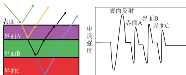
图4 时域成像剖面示意图
