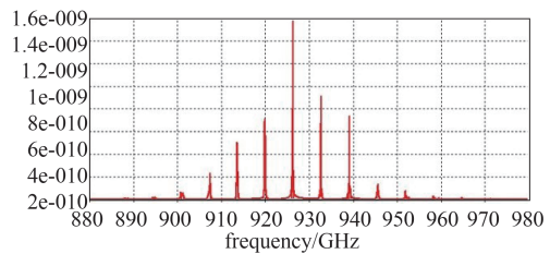
Fig. 16 FFT spectrum analysis with voltage of 11.7 kV 图 16 11.7 kV 同步电压快速傅里叶频谱分析
