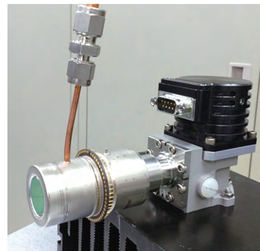
图 1 II 类超晶格长波红外探测器杜瓦组件
