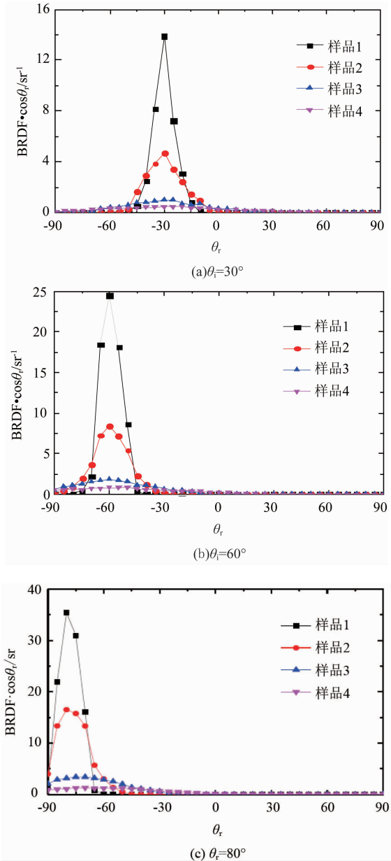
图3 非偏振光入射时不同表面粗糙度下钛合金的 DRDF · cos \theta_r 分布 Fig.3 DRDF · cos \theta_r of titanium alloy with different surface roughness under unpolarized light incidence
