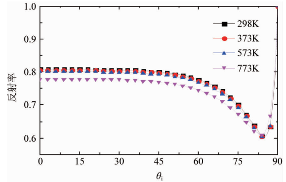
图 1 非偏振光入射时不同温度下光滑钛合金平板的反射率
