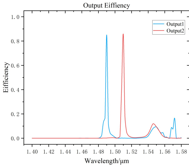
图4 初始模型的滤波性能仿真
