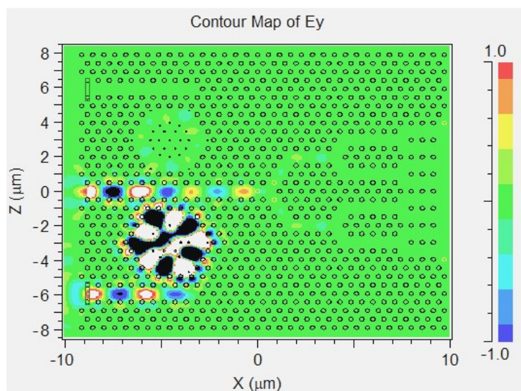
图10 1.510\mu\text{m} 波长滤波结构光场分布
