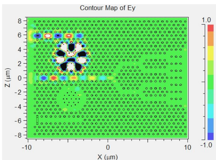
图9 1.490\mu\text{m} 波长滤波结构光场分布
