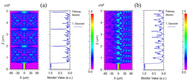
Fig. 2 Simulation of light field. : (a) Linear NCF; (b) Curved NCF 图2 光场模拟仿真图.: (a) 直线型NCF; (b) 弯曲线NCF
